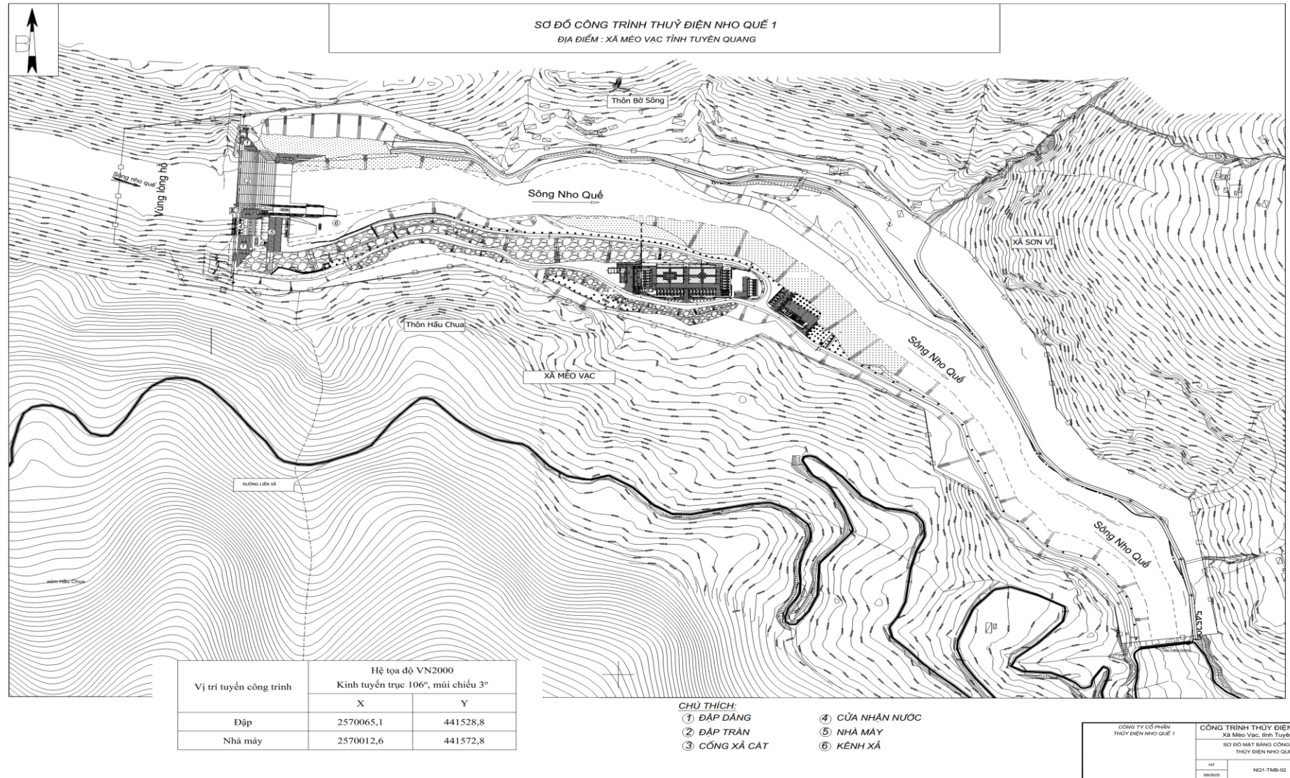
Hình 2: Sơ đồ mặt bằng công trình thủy điện Nho Quế 1
