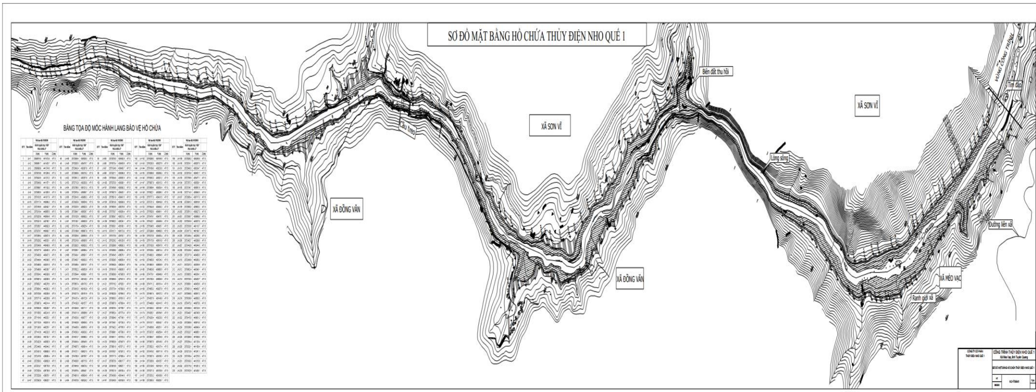
Hình 3: Sơ đồ mặt bằng khu vực hồ chứa thủy điện Nho Quế 1
